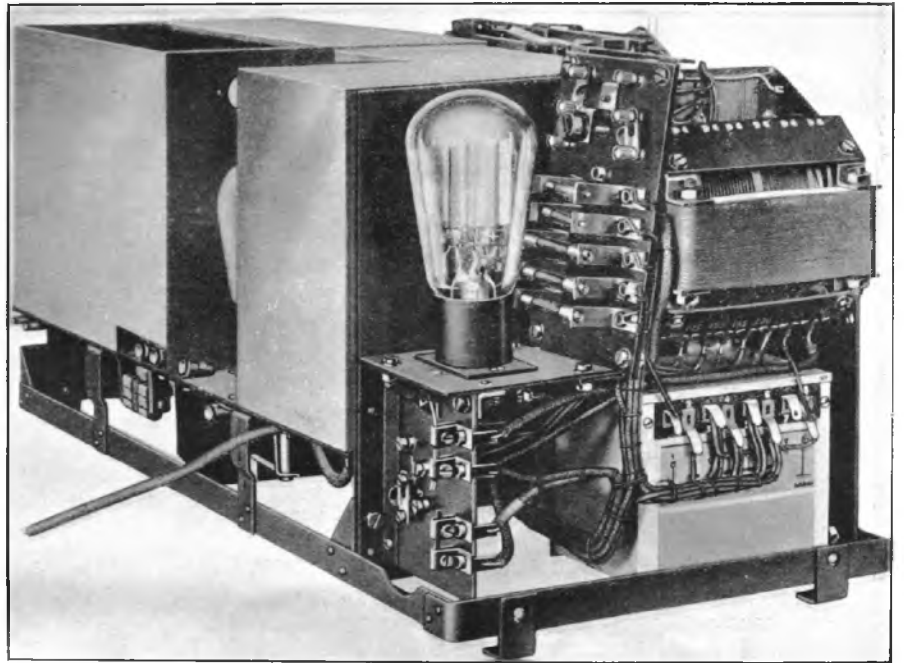
BOVEN- EN ZIJAAZICHT VAN HET INWENDIGE DER „T 40 W”
