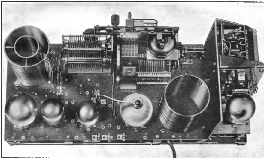
BOVEN- EN ZIJAAZICHT VAN HET INWENDIGE DER „T 40 W”
