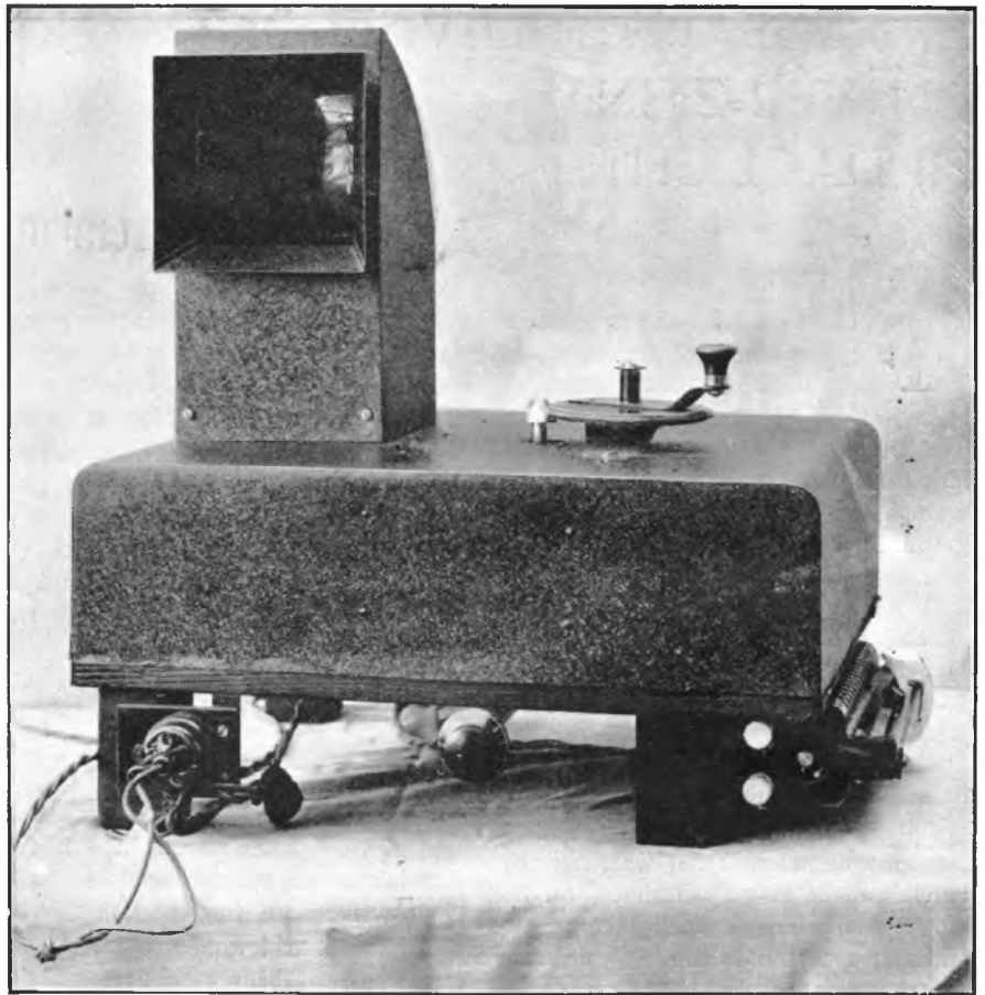
De Mihaly „daglicht”-televisieontvanger. Het beeld verschijnt in de opening links boven.
