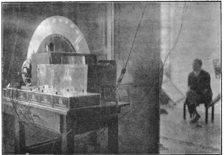
De Mihaly daglichtzender in bedrijf.
